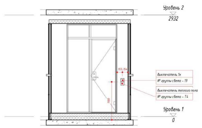
2 Фасад 33 - а 1:40
