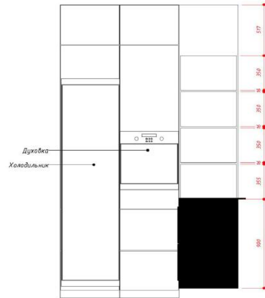
3 Узел 17 1:25
