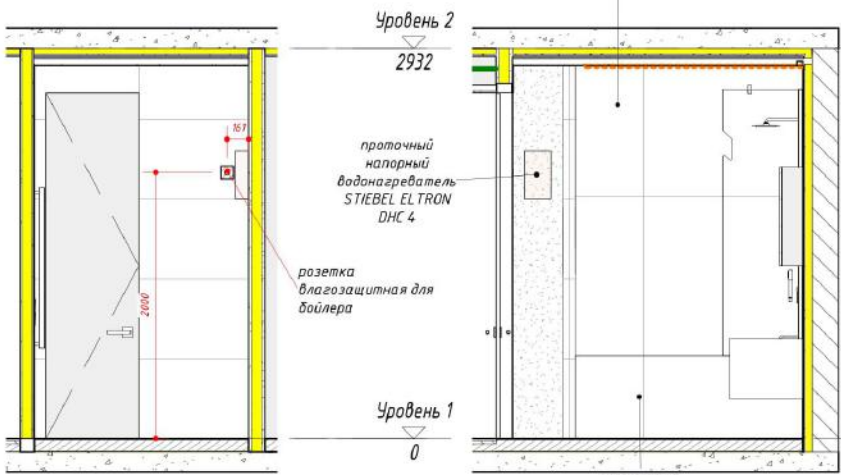
1 Фасад 1 - а 1: 40
