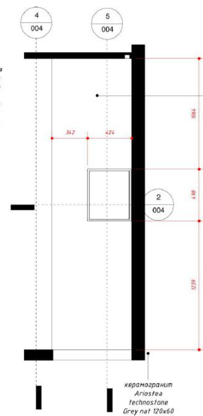
3 Узел 5 1:25
