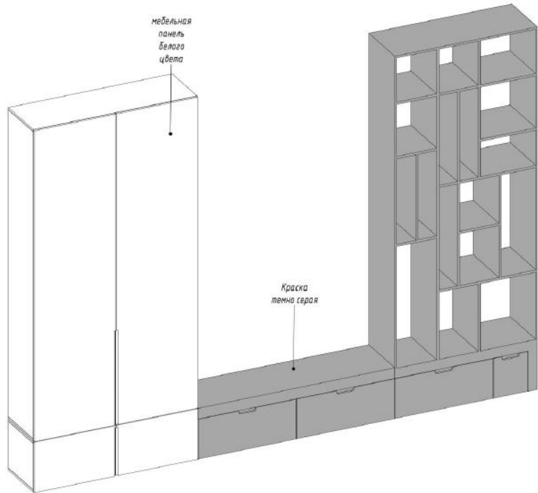
1 3D орто
