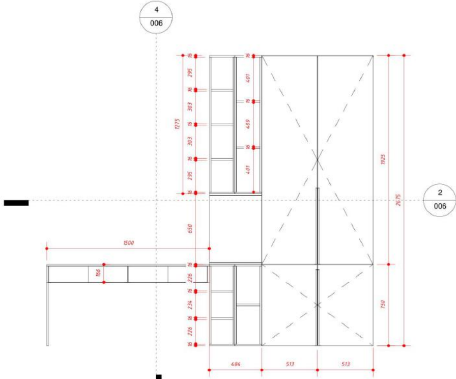
3 Узел 0 1:25
