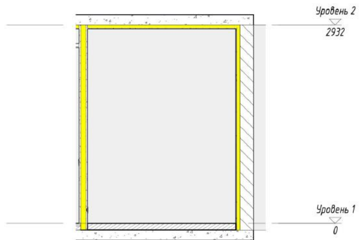
1 Фасад 27 - а 1:40
