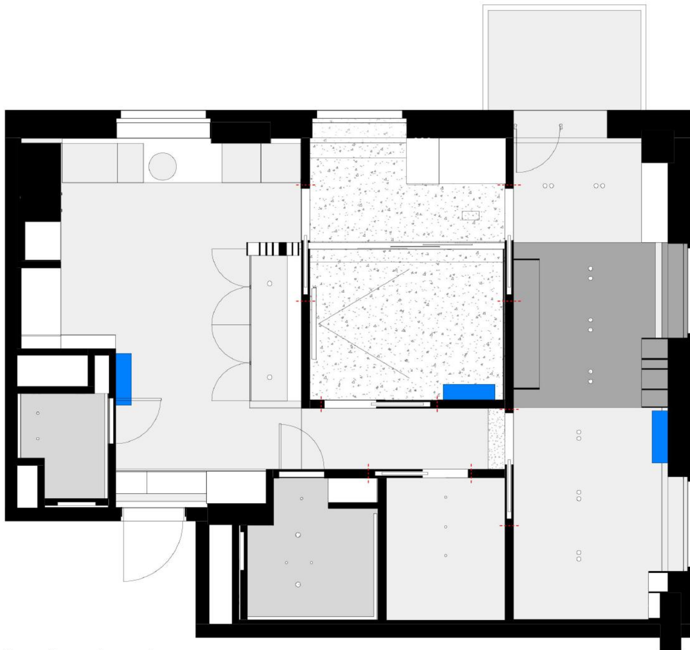
1 План привязки кондиционеров 1:40
