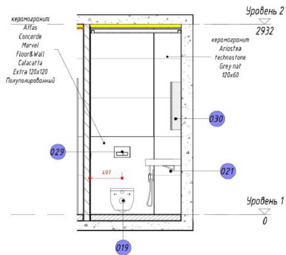
3 Фасад 7 - а 1:40
