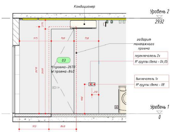
4 Фасад 36 - а 1:40
