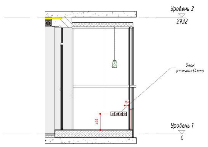
1 Фасад 32 - а 1:40
