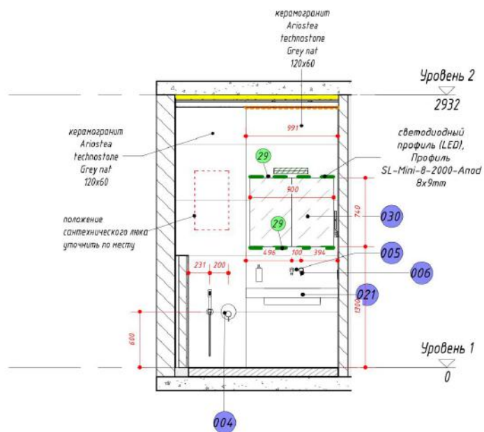
2 Фасад 6 - а 1:40
