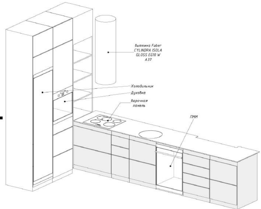
3 Узел 17 1:25
