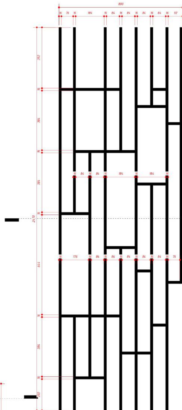
3 Узел 12 1 : 10
